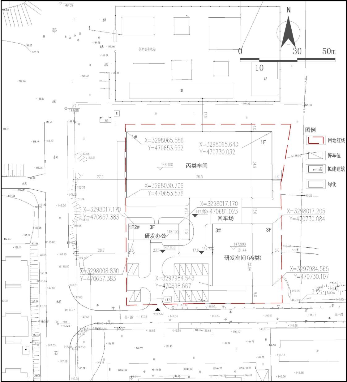
原厂区总平面图
